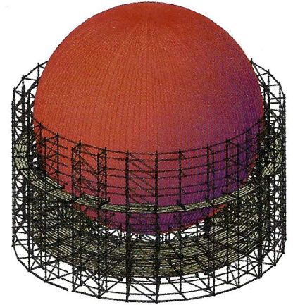
ESFERA EXTERIOR
